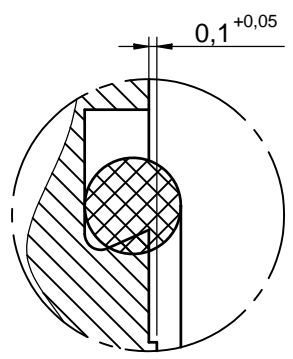
detail A 15:1
