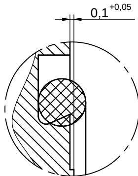
detail A 15:1
