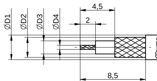
Kabelzuschnitt / stripping dimension
