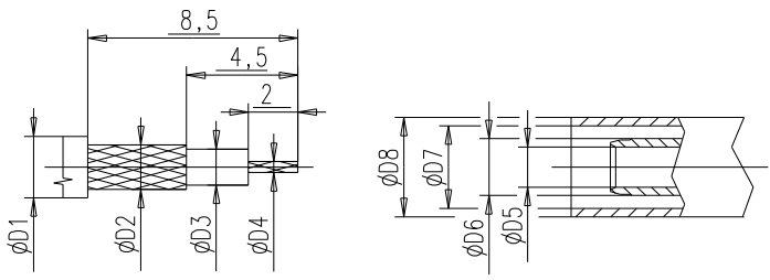
Kabelzuschnitt Stripping dimension
