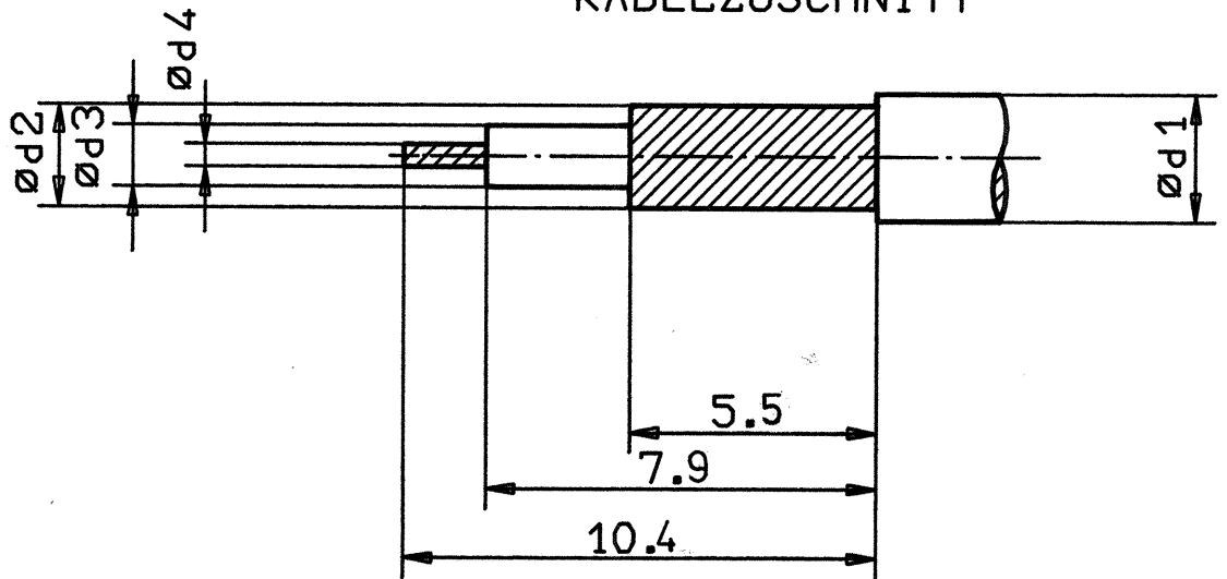
FUER KABEL
